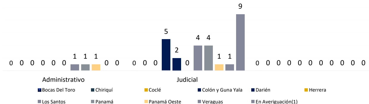
Gráfica 8. NÚMERO DE COLABORADORES INVESTIGADOS, POR ÁREA DE TRABAJO, SEGÚN PROVINCIA: DEL 1 DE ENERO AL 28 DE FEBRERO DE 2022.
