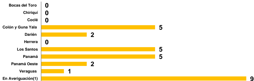
Gráfica 5. NÚMERO DE COLABORADORES INVESTIGADOS SEGÚN PROVINCIA: DEL 1 DE ENERO AL 28 DE FEBRERO DE 2022.
