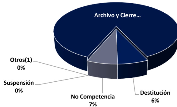
Gráfica 9. DISTRIBUCIÓN PORCENTUAL DE LOS TIPOS DE SALIDAS DE LOS EXPEDIENTES POR COLABORADOR, SEGÚN MIEMBRO SUSTANCIADOR QUE LO INVESTIGA, POR DECISIÓN DEL CASO: DEL 1 DE ENERO AL 28 DE FEBRERO DE 2022.
