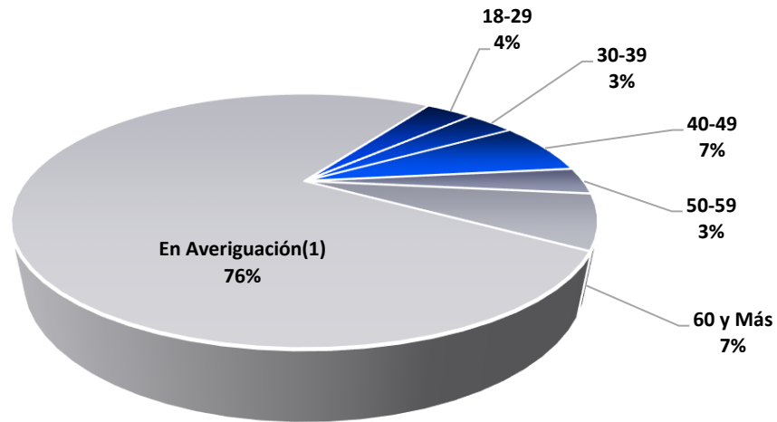
Gráfica 4. DISTRIBUCIÓN PORCENTUAL DE LOS COLABORADORES INVESTIGADOS, SEGÚN RANGO DE EDAD: DEL 1 DE ENERO AL 28 DE FEBRERO DE 2022.
