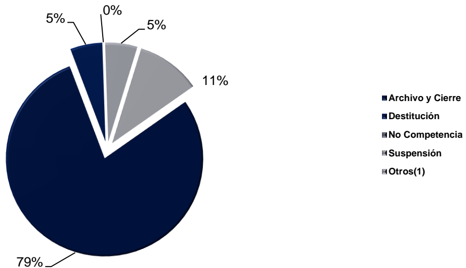
Gráfica 2. DISTRIBUCIÓN PORCENTUAL DE LAS SALIDAS DE LOS EXPEDIENTES QUE MANTIENE EL CONSEJO DISCIPLINARIO SEGÚN TIPO: DEL 1 DE ENERO AL 28 DE FEBRERO DE 2022.
