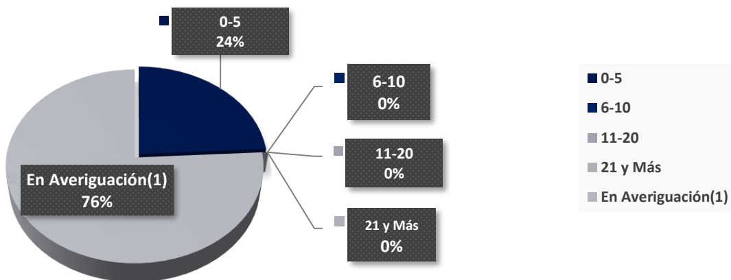
Gráfica 7. DISTRIBUCIÓN PORCENTUAL DE LOS COLABORADORES INVESTIGADOS, SEGÚN RANGO DE TIEMPO DE LABOR EN LA INSTITUCIÓN, POR RANGO DE TIEMPO EN EL PUESTO DONDE REALIZA LA FALTA: DEL 1 DE ENERO AL 28 DE FEBRERO DEL 2022
