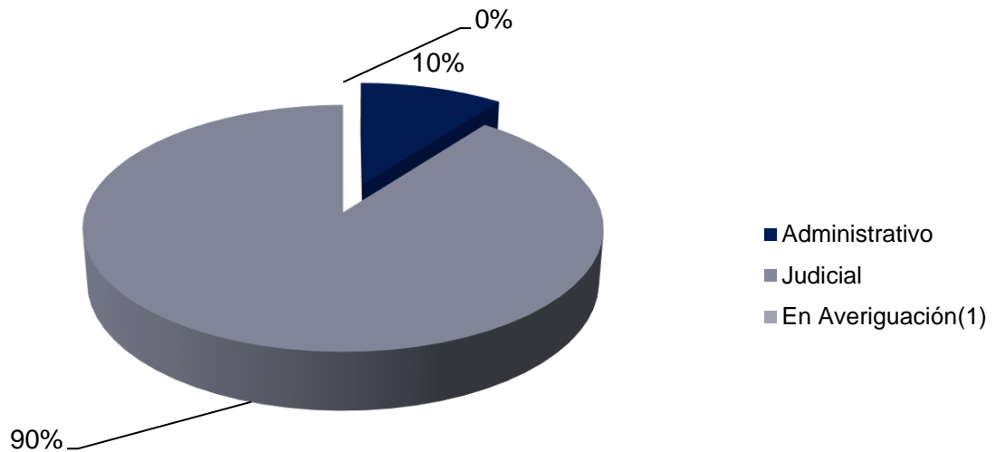
Gráfica 3. DISTRIBUCIÓN PORCENTUAL DE LOS COLABORADORES INVESTIGADOS POR EL CONSEJO DISCIPLINARIO SEGÚN TIPO: DEL 1 DE ENERO AL 28 DE FEBRERO DE 2022.
